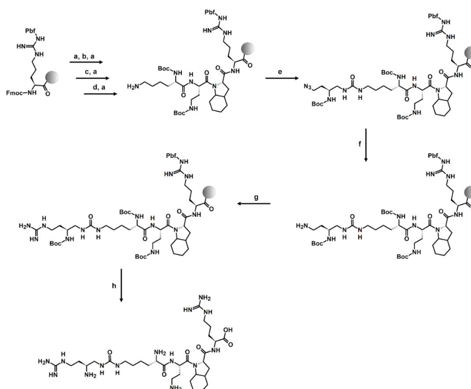
Scheme 1. The solid-phase peptide synthesis (SPPS) strategy on the example of urea–peptide hybrid 4 : (a) 20% piperidine in DMF; 20 min; (b) 2 eq Fmoc-Oic-OH, 2 eq HCTU, 5 eq DIPEA, 90 min; (c) 2 eq Fmoc-Dab(Boc)-OH, 2 eq HCTU, 5 eq DIPEA, 90 min; (d) 2 eq Boc-Lys(Fmoc)-OH, 2 eq HCTU, 5 eq DIPEA, 90 min; (e) 1.5 eq Boc-Dab(N 3 ) BB, 3 eq DIPEA, 50 W, 60 °C, 2 × 15 min; (f) 10 eq 1 M PMe 3 /THF, 7:3 1,4-dioxane:H 2 O, 50 W, 60 °C, 2 × 30 min; (g) 5 eq DMPCN, 19.5 eq DIPEA, 7 days; (h) 95:2.5:2.5 TFA:H 2 O:TIS, 3 h.
