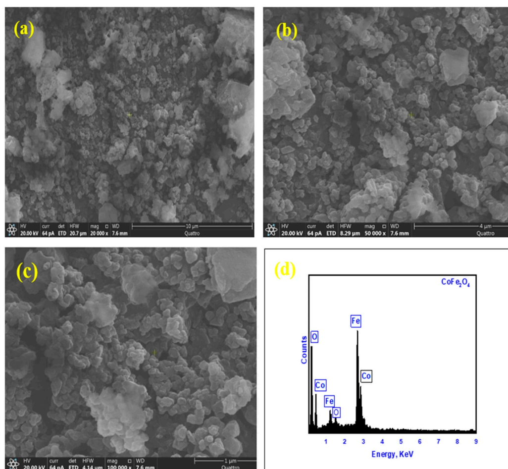
Figure 4. SEM images (a–c), (d) EDX spectrum of \text{CoFe}_2\text{O}_4 nanoparticles.
