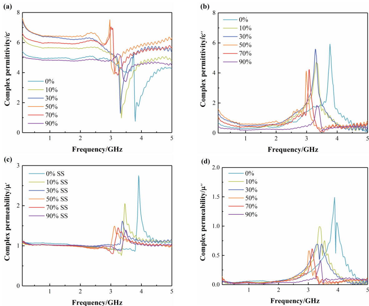
Figure 12. Electromagnetic parameters of AAS with different SS dosages (a) \epsilon' ; (b) \epsilon'' ; (c) \mu' ; (d) \mu'' .
