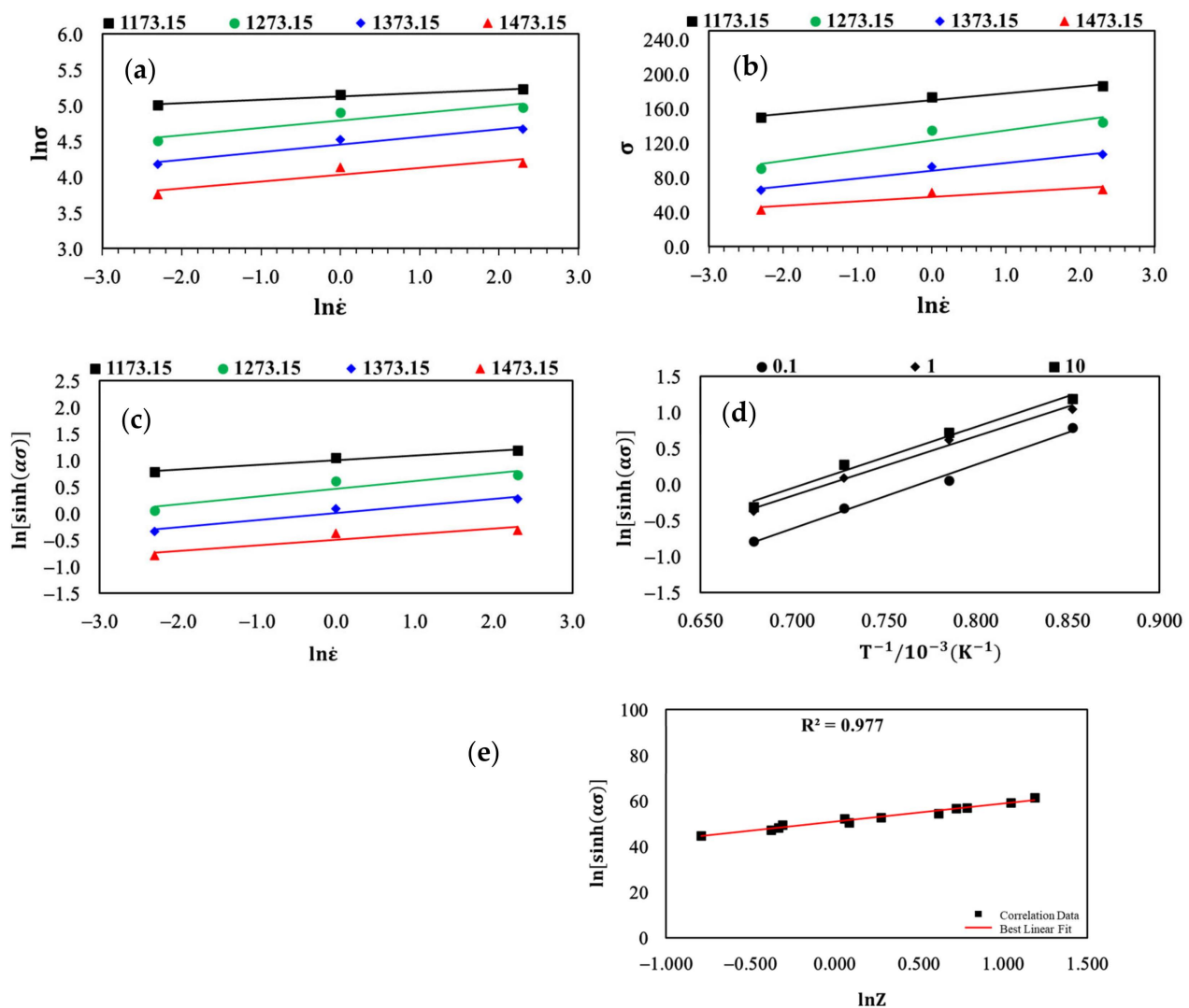
Figure 3. Plots between (a) \sigma - \ln \dot{\epsilon} ; (b) \ln \sigma - \ln \dot{\epsilon} ; (c) \ln[\sinh(\alpha \sigma)] - \ln \dot{\epsilon} ; (d) \ln[\sinh(\alpha \sigma)] - 1000/T ; and (e) \ln[\sinh(\alpha \sigma)] - \ln Z .
