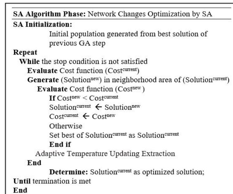
Figure 8. SA Algorithm pseudocode.
